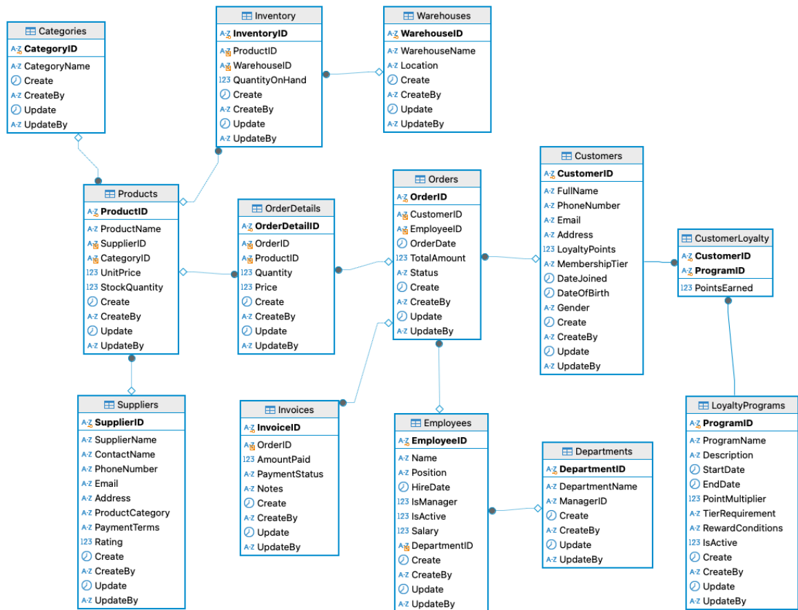
Hình 1: Relationship của các bảng trong hệ thống ERP
